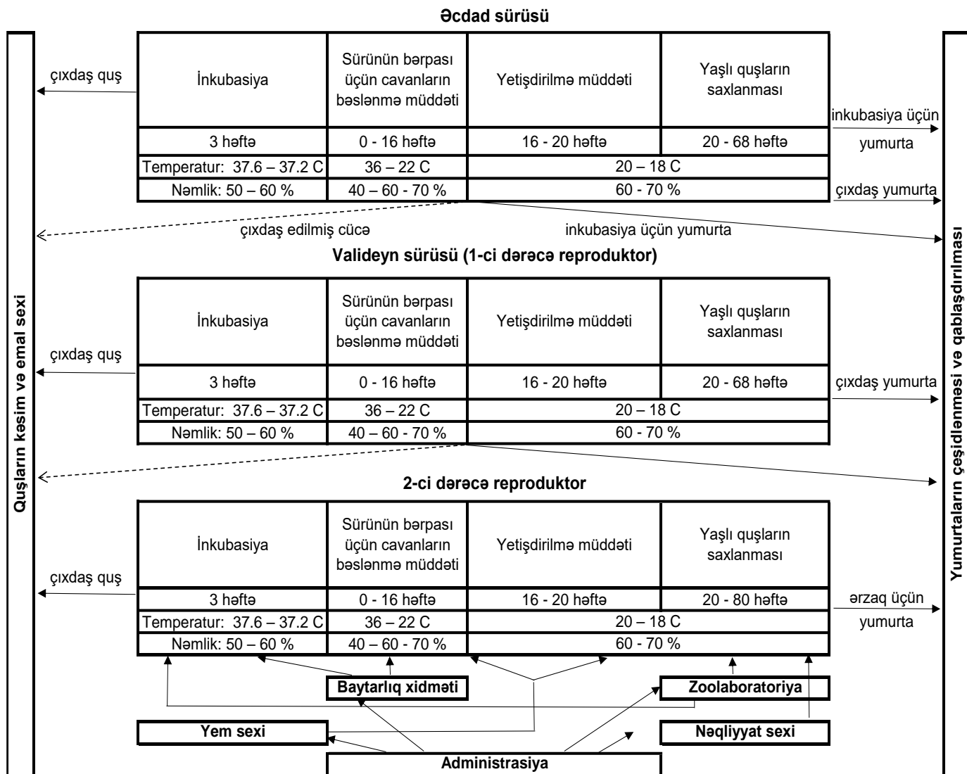
Sxem 1. Damazlıq yumurta istehsalı üzrə texnoloji prosesin təsviri
